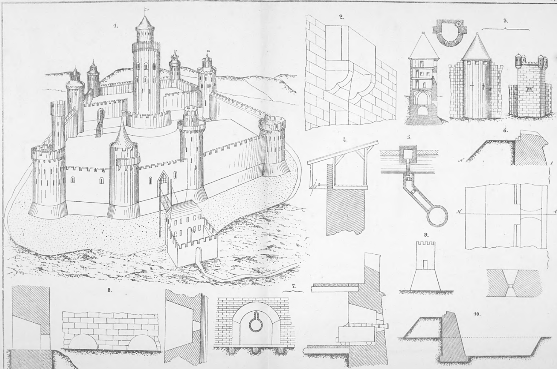
1, Башня съ болотономъ. - 2, Мушкетъри. - 3, Башни. - 4, Надстройки въ горескихъ оградахъ. - 5, Бастионъ и барбаканъ. - 6, Амбразури въ брустверъ. - 7, Амбразури. - 8, Оборона подошвы стѣны. - 9, Вартени. - 10, Камениый брустверъ. -
