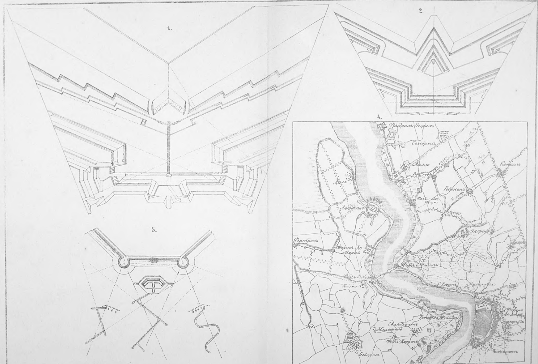
1 - Система Спелле. 2, Нидерландская система укреплений. 3, Атака крепости. 4, Осада Антверпена. 1584 года. 5, Атака крепости.
